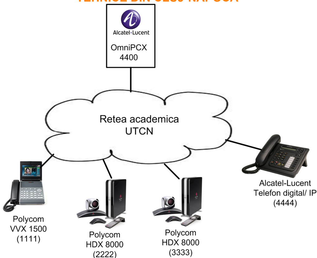
Figura 1. Schema bloc
